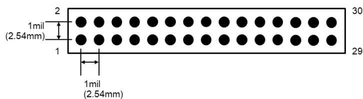
図 3 CN2 スルーホール形状
