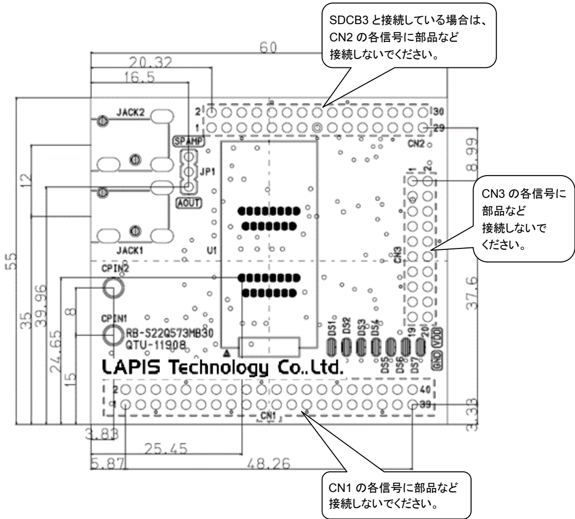
図 5 配置図
