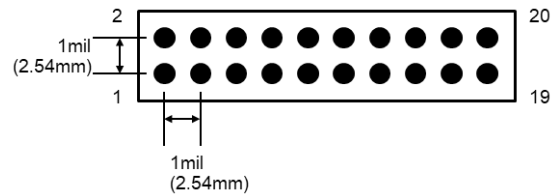
図 4 CN3 スルーホール形状
