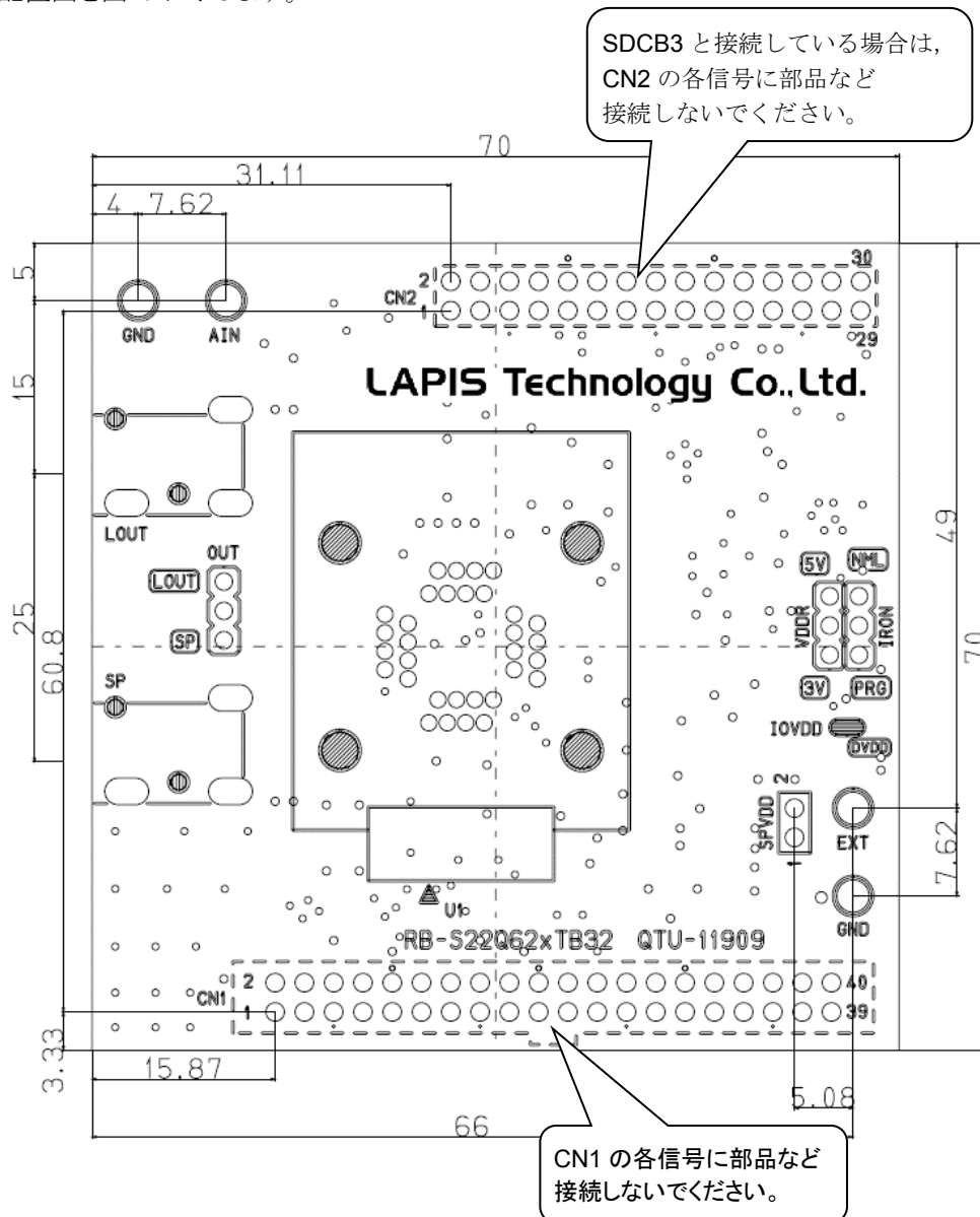
図 7 配置図
