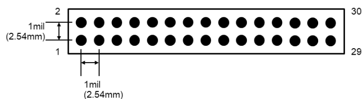
図 6 CN2 スルーホール形状
