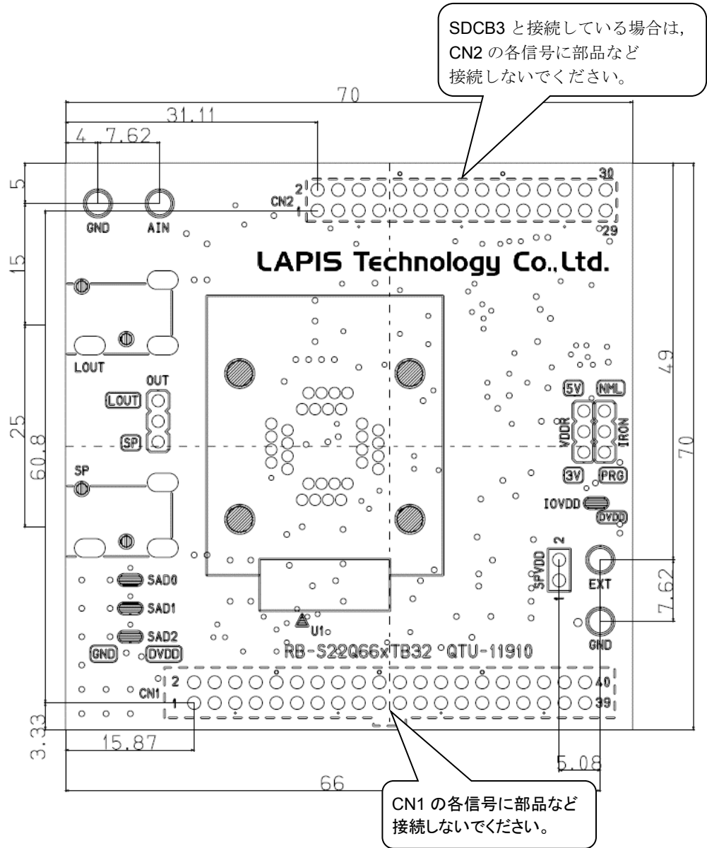
図 8 配置図
