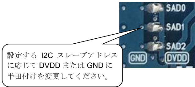
図 4 SAD2-0 ランド
