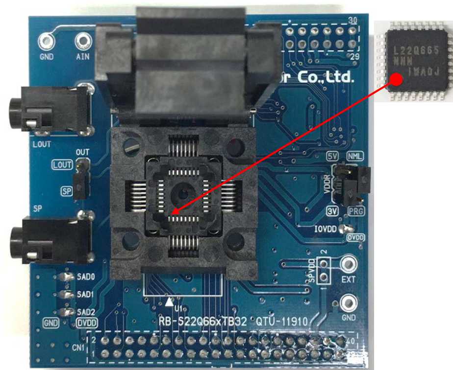
図 1 外観
