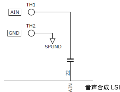
図 2 AIN スルーホール
