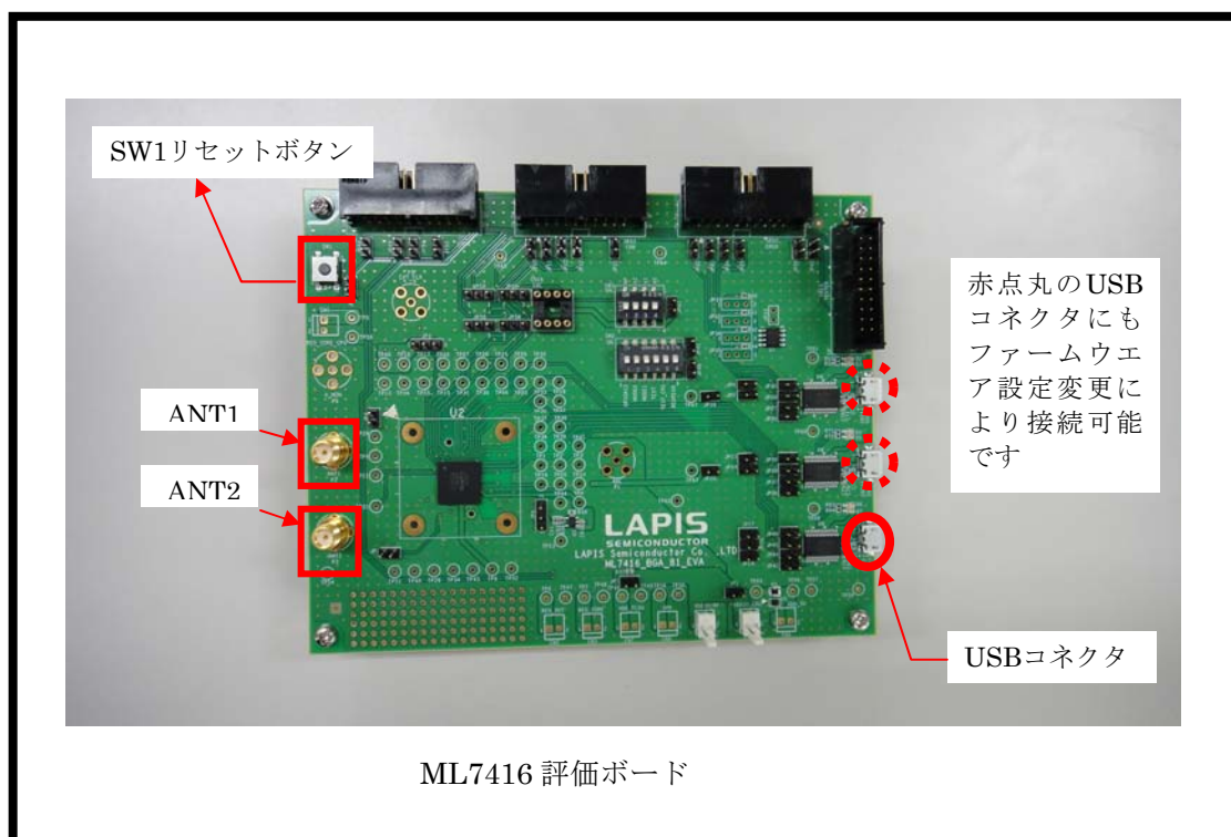
図 1: 評価ボードと USB ケーブルの接続
