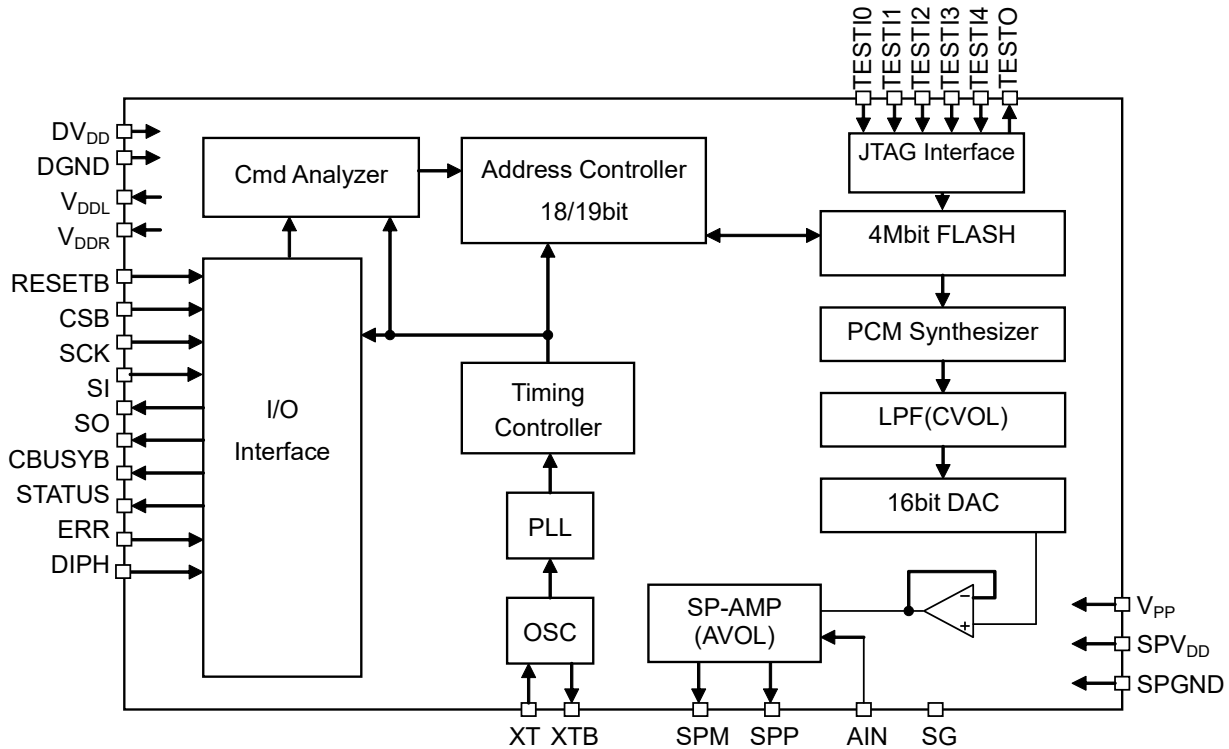
ML22Q563-NNN/ML22Q563-xxx ブロック図
