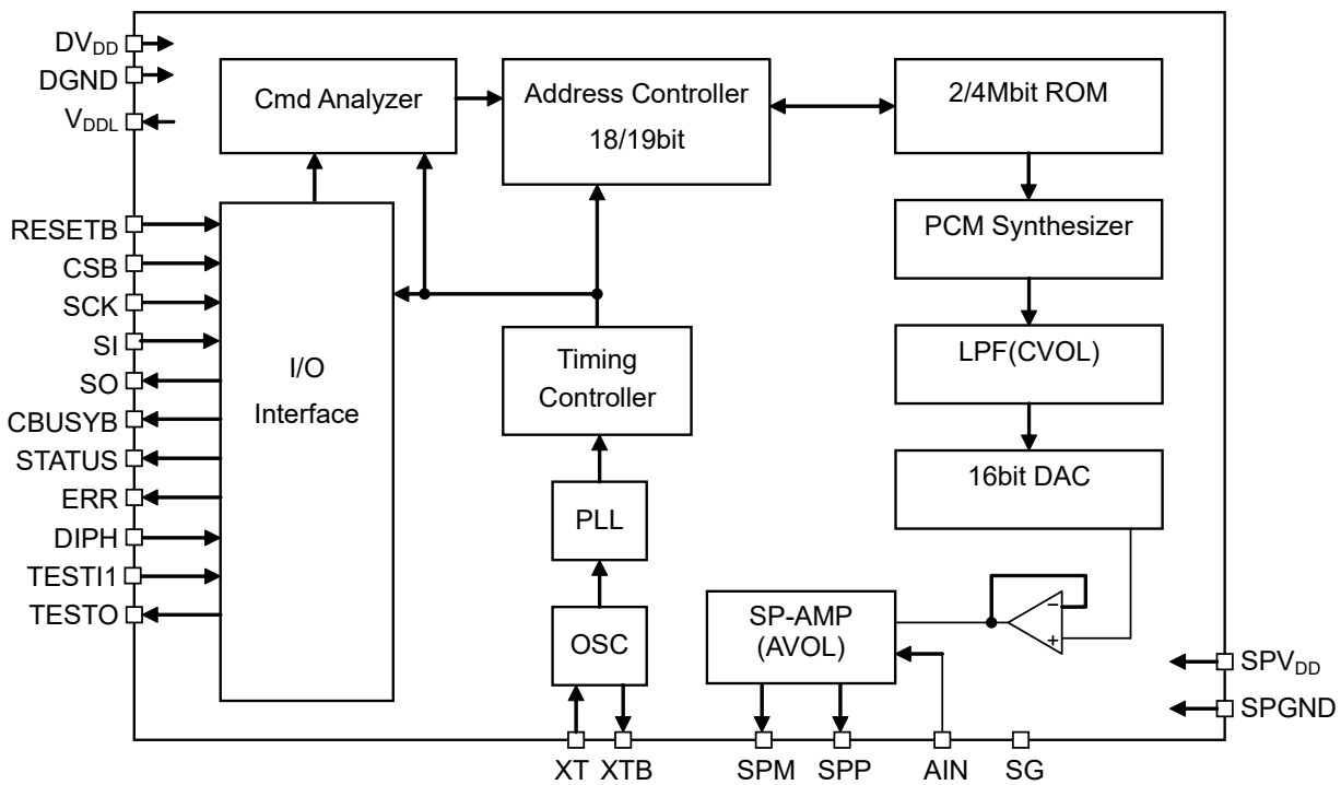
ML2256X-xxx ブロック図
