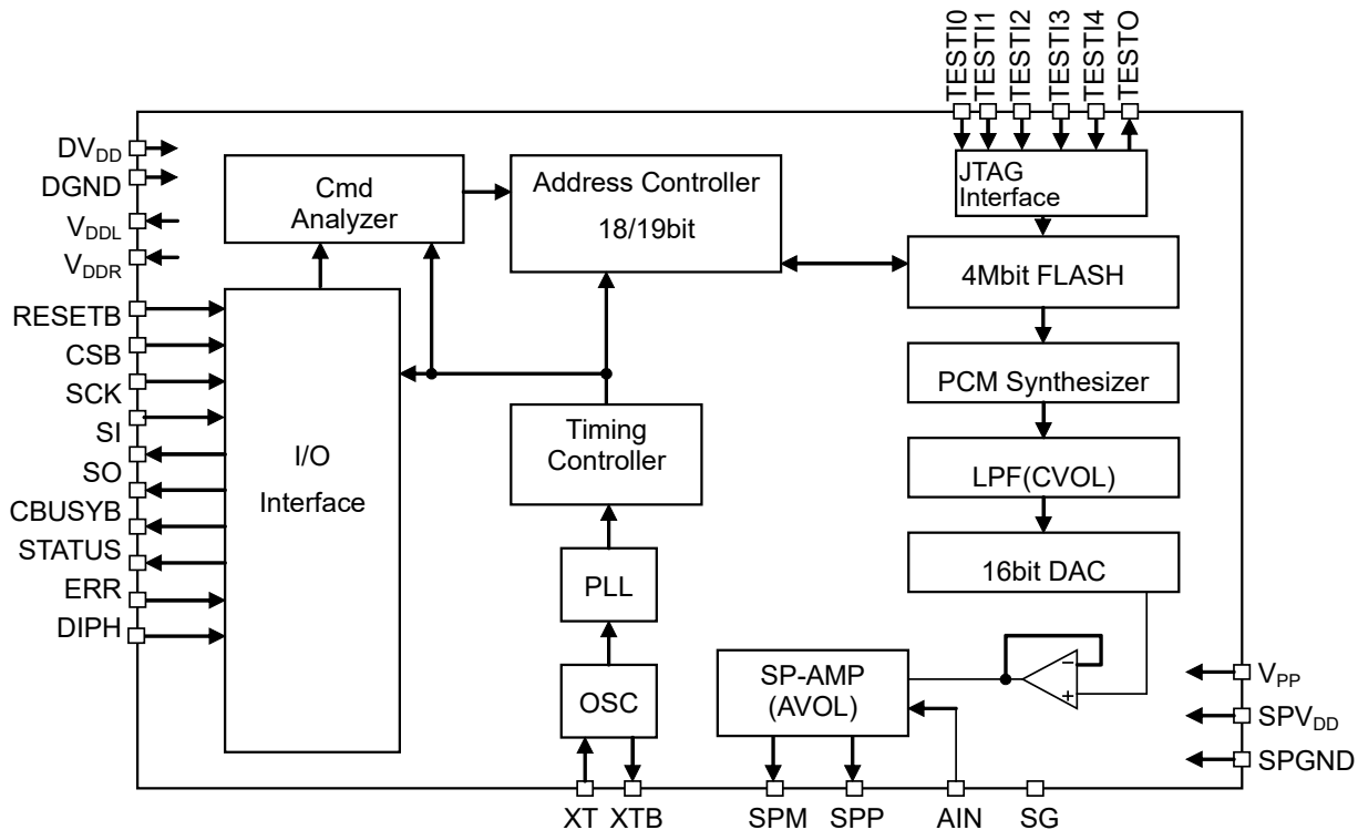
ML22Q573-NNN/ML22Q573-xxx ブロック図
