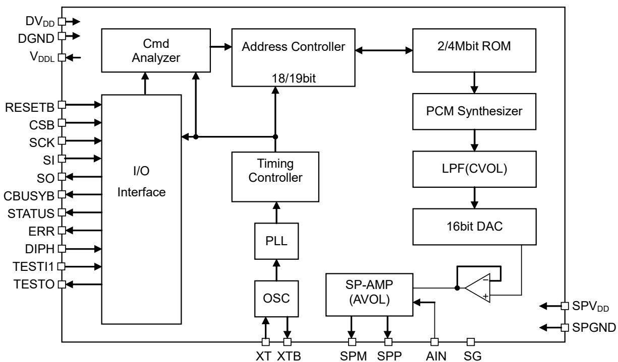
ML2257X-xxx ブロック図
