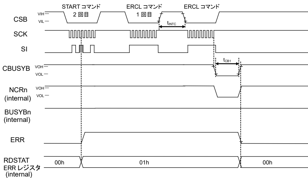
2 回コマンド入力モードエラー時タイミングチャート
