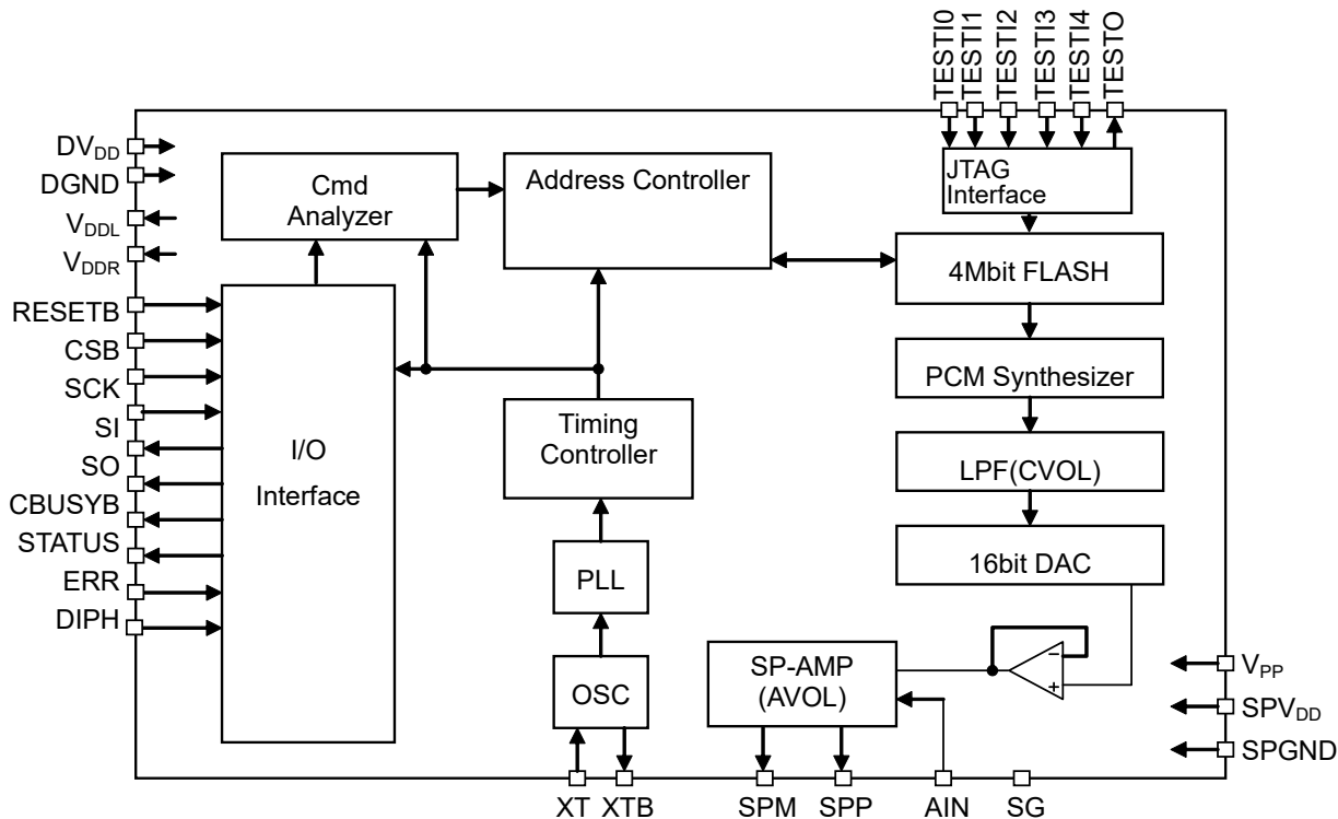
ML22Q553-NNN/ML22Q553-xxx ブロック図
